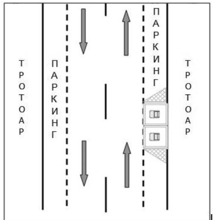
Слика 20: Постављање подземног контејнера на делу коловозне површине намењене за паркирање
