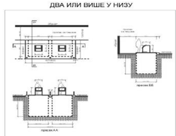
Слика 23: Шематски приказ типа Ц
