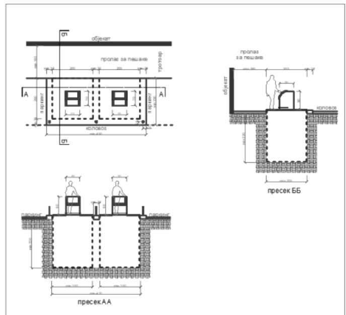
Слика 22: Шематски приказ типа Ц
