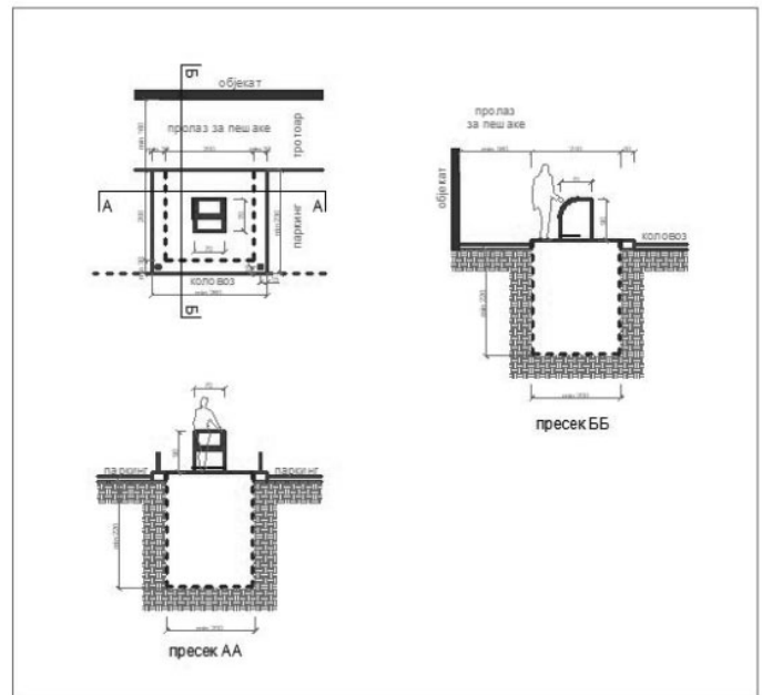
Слика 21: Шематски приказ типа Б
